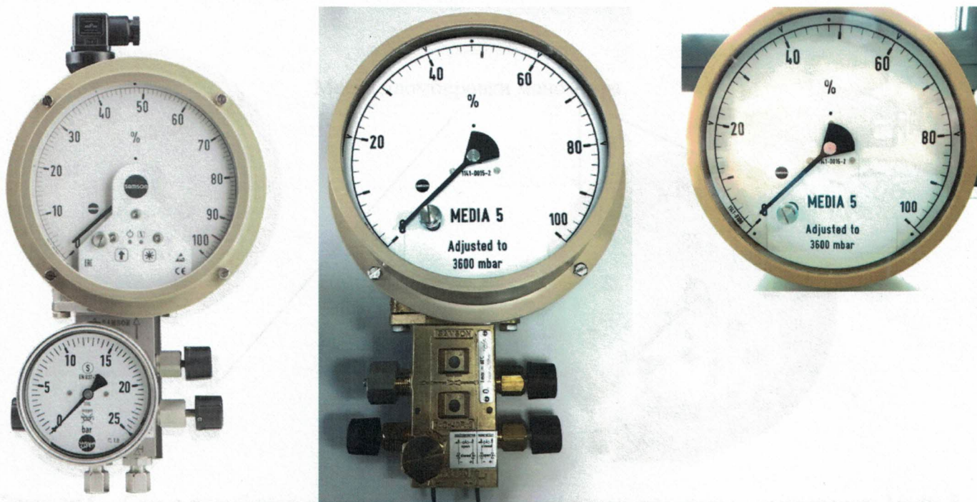
Рисунок 2 - Общий вид манометров дифференциальных показывающих Media 5
